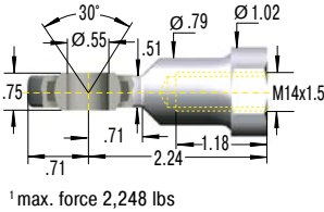
E14 Swivel Eye DIN 648
